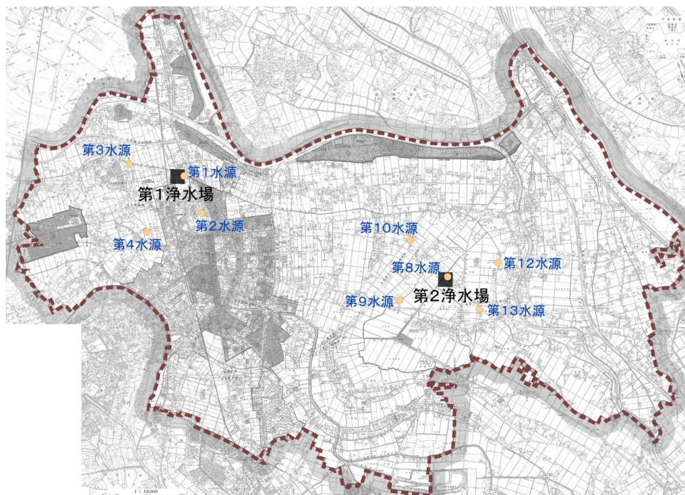
給水区域と施設位置図
