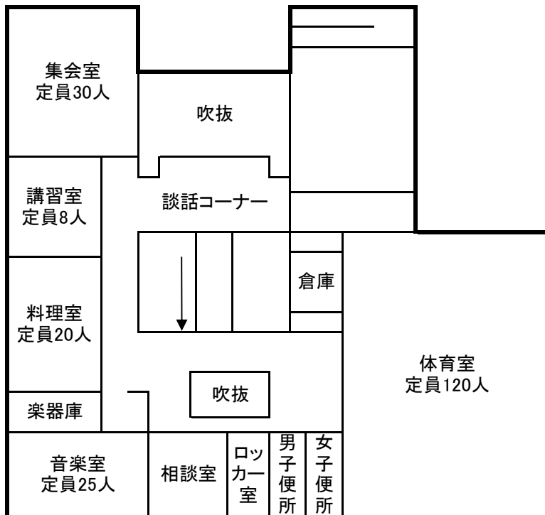
2階（勤労青少年ホーム）平面図
