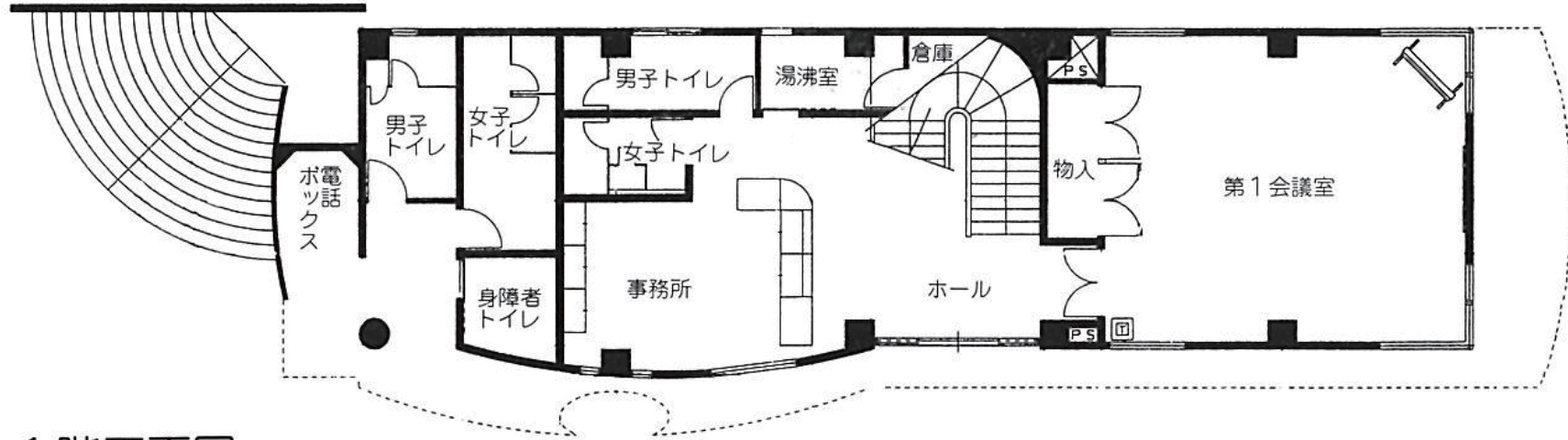
1階平面図
