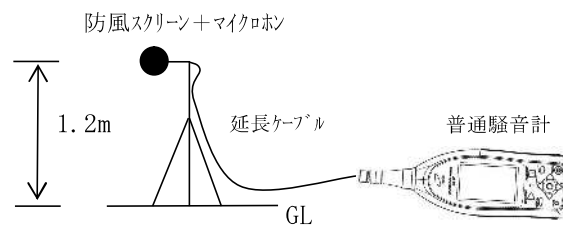
図 3.4.1 測定機器接続図
