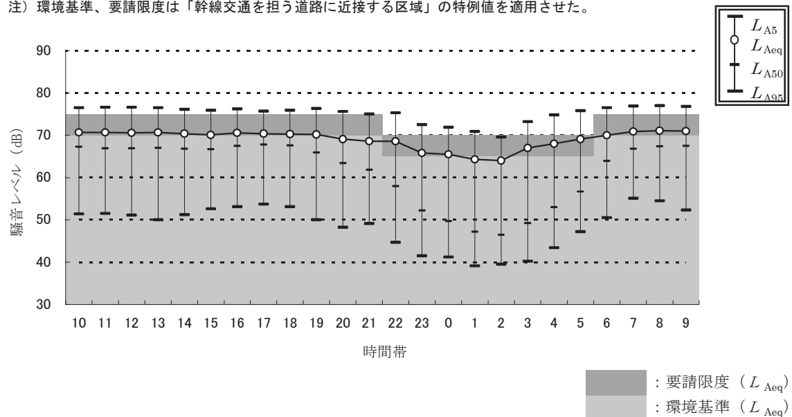
図 3.5.1 騒音時間変化グラフ
