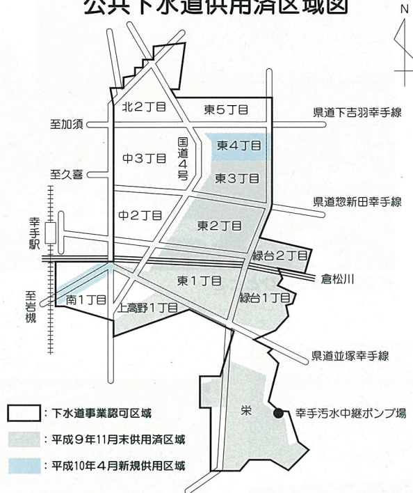
公共下水道供用済区域図
