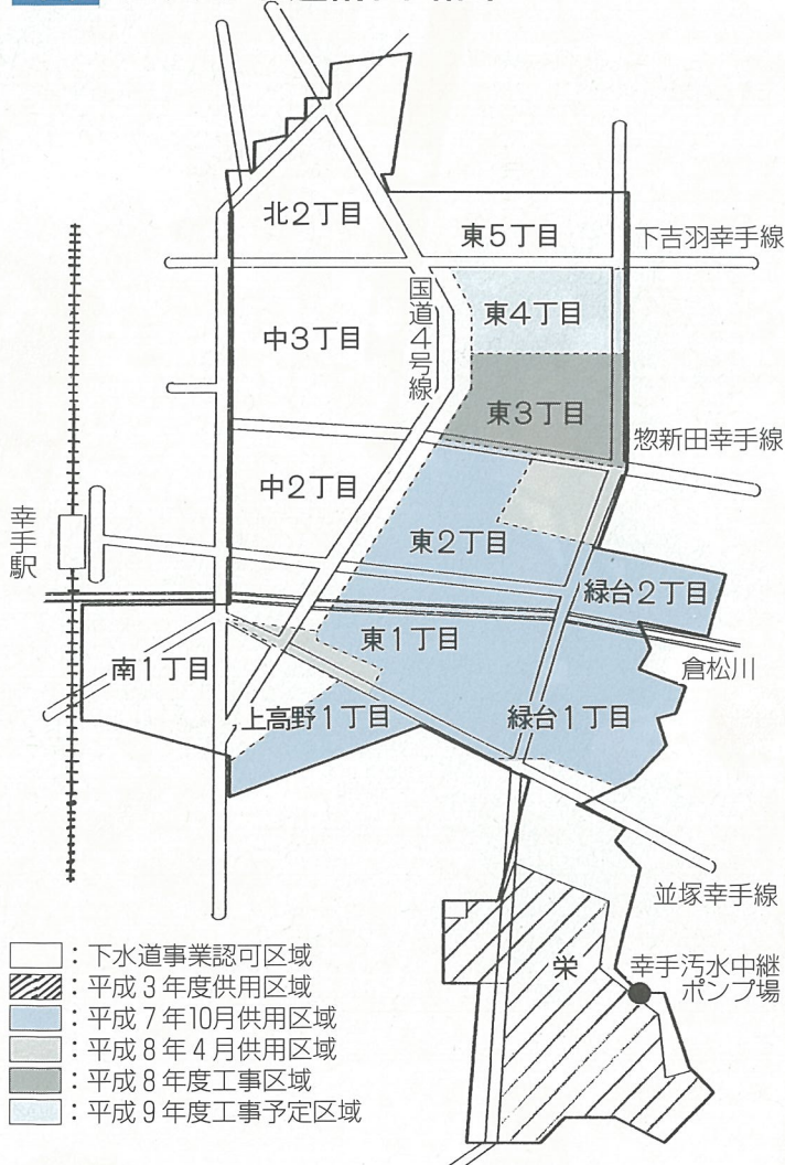
公共下水道計画略図
