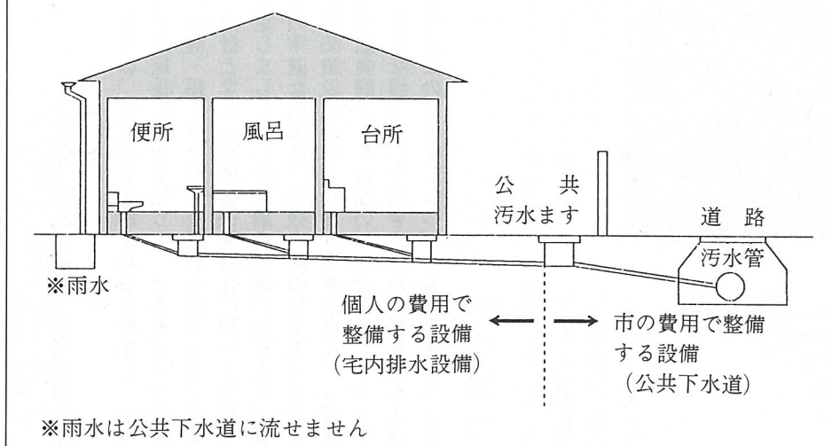
宅内排水設備図
